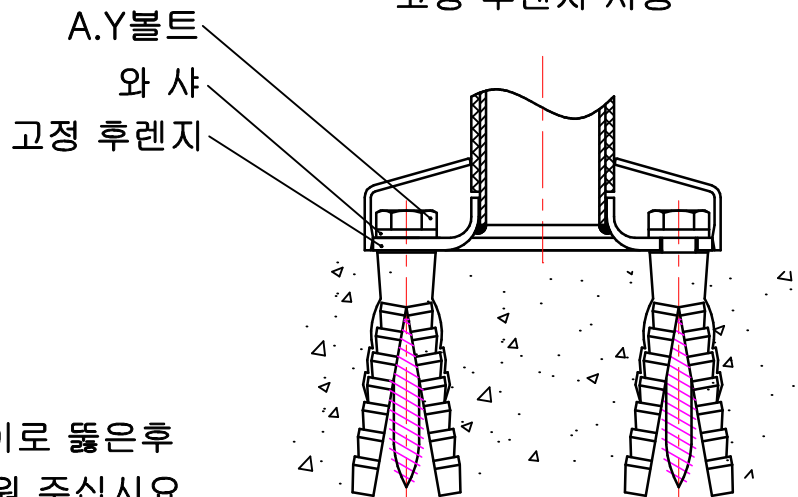
고정 후렌지 시공
